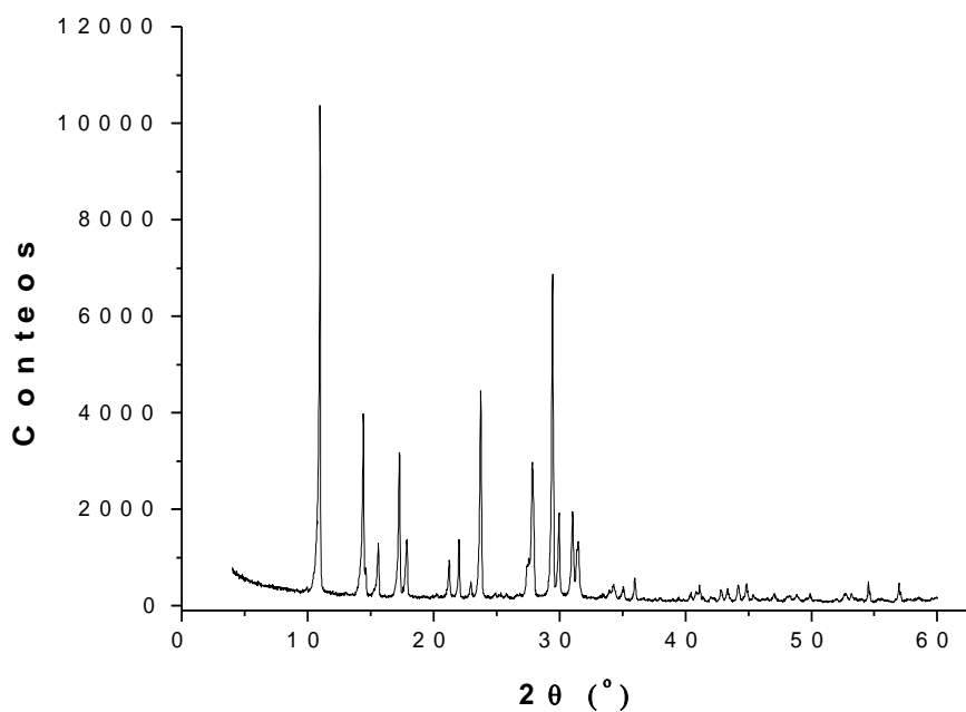
Fig. 2. Patrón de difracción de Rayos X del compuesto N-furoil-O-etil-S-metilcarbonimidotioato.
